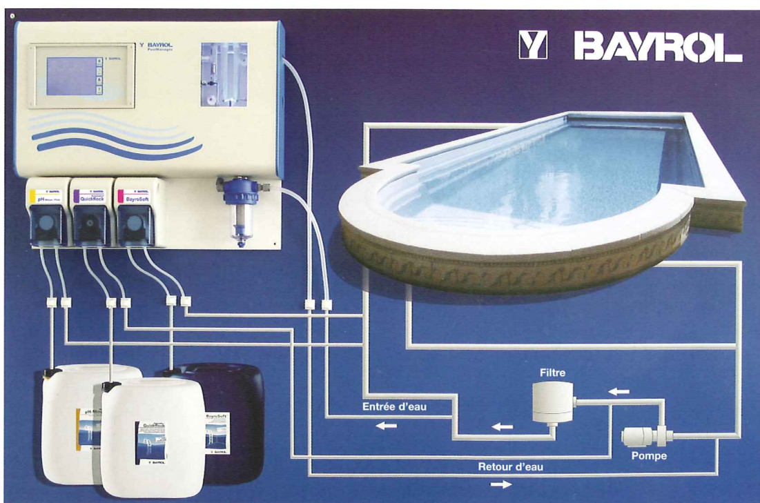
Raccordement du PoolManager Oxygène Actif
